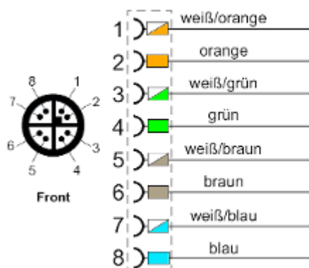
M12-Buchse
